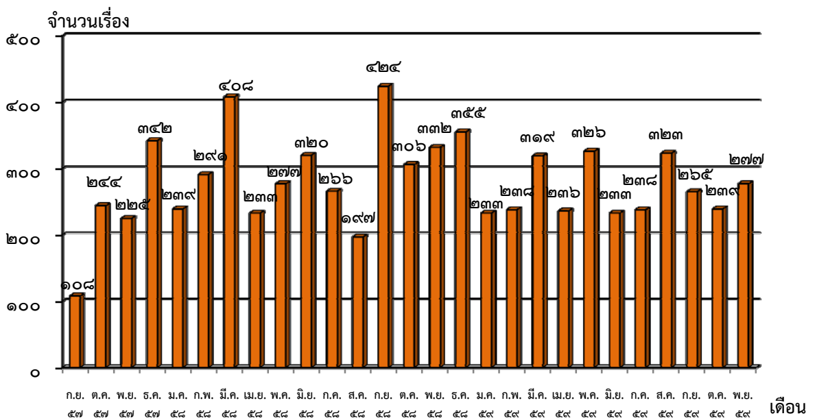
แผนภูมิแสดงจำนวนมติคณะรัฐมนตรีในช่วงตั้งแต่ ๑๖ กันยายน ๒๕๕๗ - ๓๐ พฤศจิกายน ๒๕๕๙
