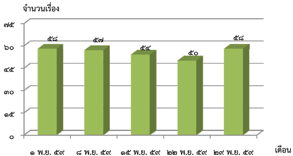
แผนภูมิแสดงจำนวนมติคณะรัฐมนตรีในเดือนพฤศจิกายน ๒๕๕๙
